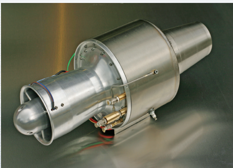
Microturbines
